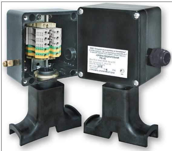
Рис. 26. РТВ 401. Соединительная коробка с устройством ввода кабеля под теплоизоляцию для подключения к силовой сети саморегулирующихся электрических нагревательных кабелей
