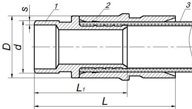
Рис. 7. Переход на сварное соединение с монтажной гильзой для труб ТВЭЛ-ПЭКС-К 1 – переход на сварное соединение; 2 – гильза (длинная); 3 – труба РЕ-Ха с армирующей системой
